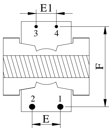
底视图
