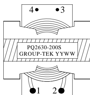
顶视图
