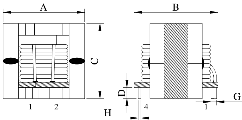
主视图
