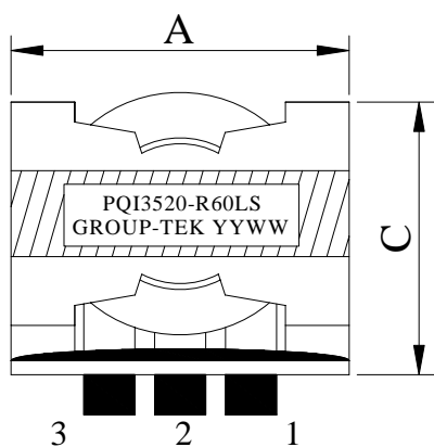
主视图
